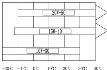
Fig. 16 Selección del lubricante.
